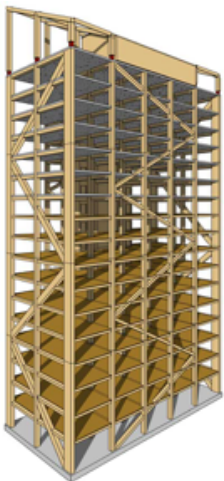
Figure 8. Maquette d'immeuble à ossature bois de grande hauteur en Norvège (Brumunddal).
